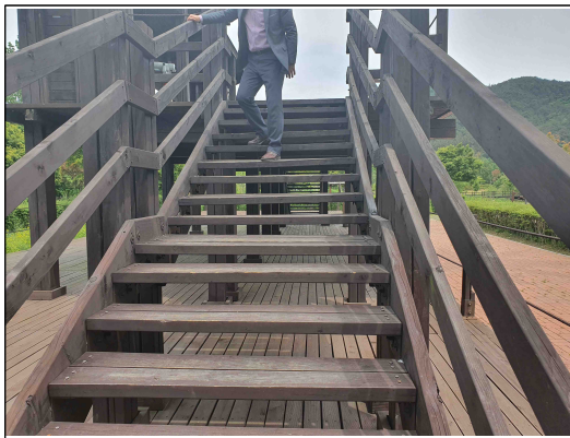
조류관찰대 계단 연결부 유동
